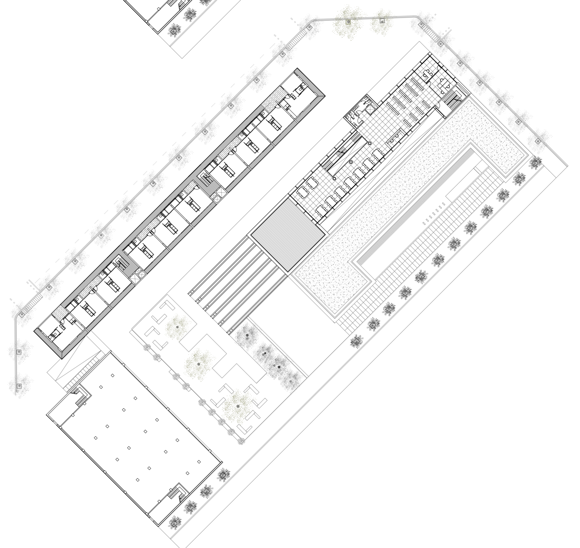
planta tipus
