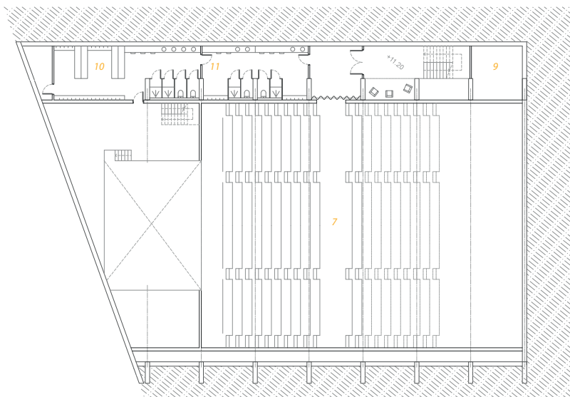
Planta soterrani; cota +11,20m
