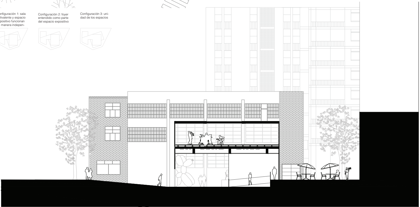
Sección transversal 1.150
