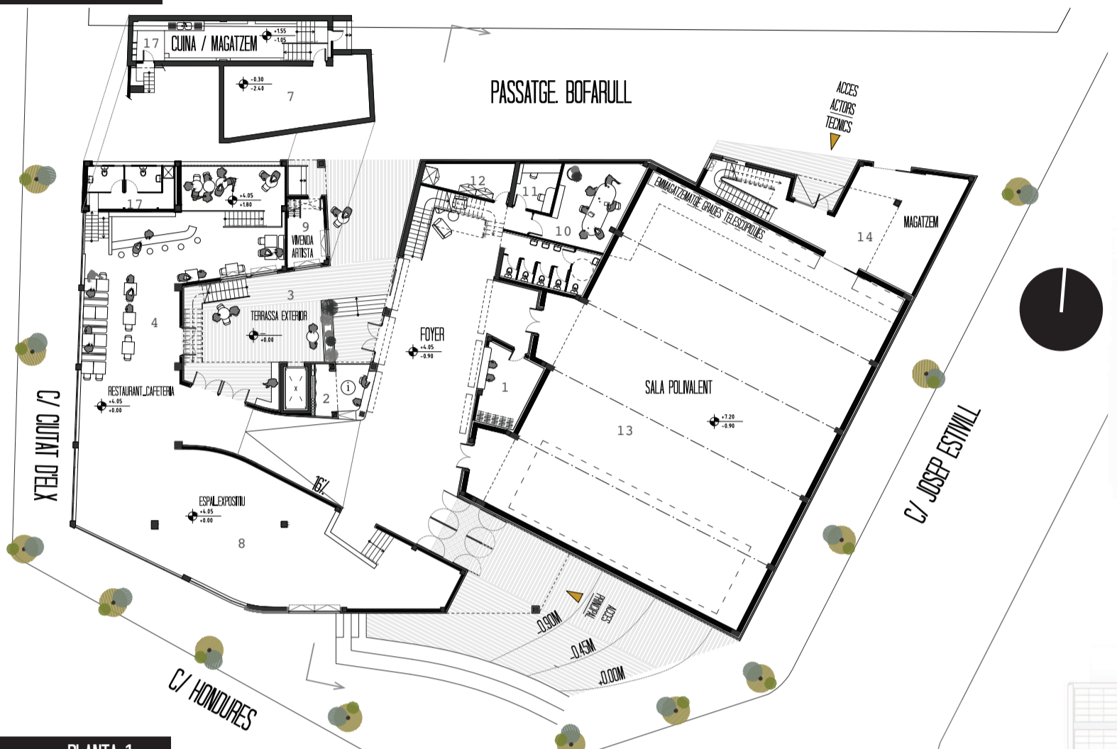
PLANTA 1 1250
