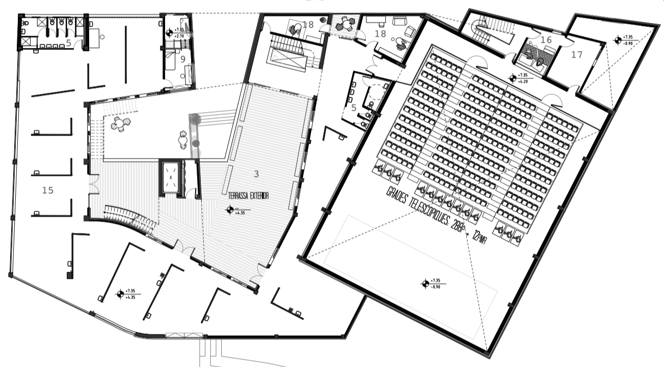
PLANTA 2 1250
